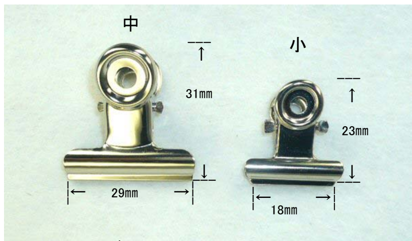
目玉クリップ
